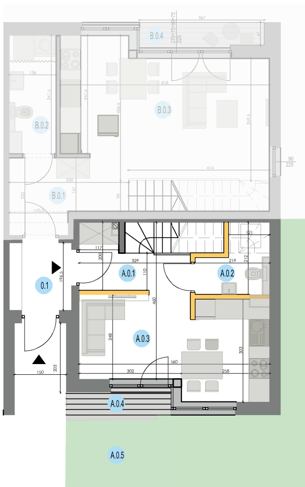
LOKAL 1A - POWIERZCHNIA UŻYTKOWA: 59,98 m 2
