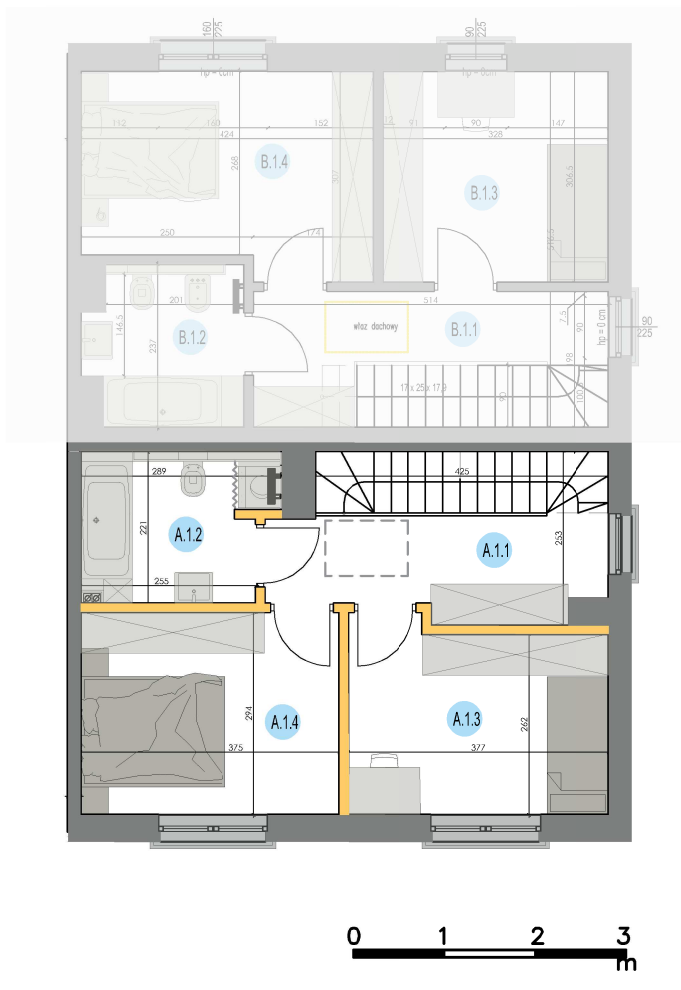
LOKAL 1A - POWIERZCHNIA UŻYTKOWA: 59,98 m 2
